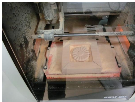
平成29年度講座の切削機による加工の様子
